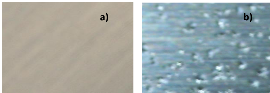
Şekil 1 (a)Paslanmaz çelik ve (b) SS/CoCr elektrotların yüzey fotoğrafları
