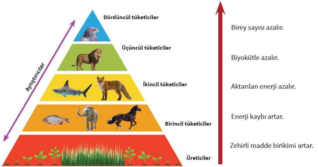
Görsel 1: Besin Zinciri ve Enerji Akışı
