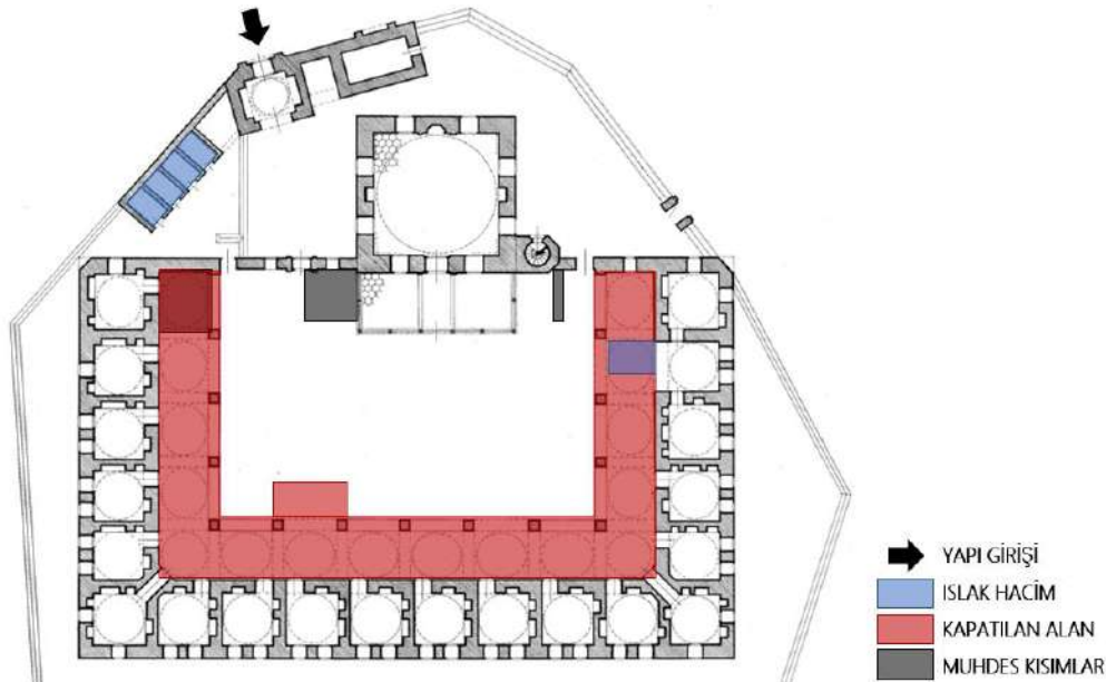
Şekil 6: Sultan Selim Medresesi Planı (Ülgen, 1939)
