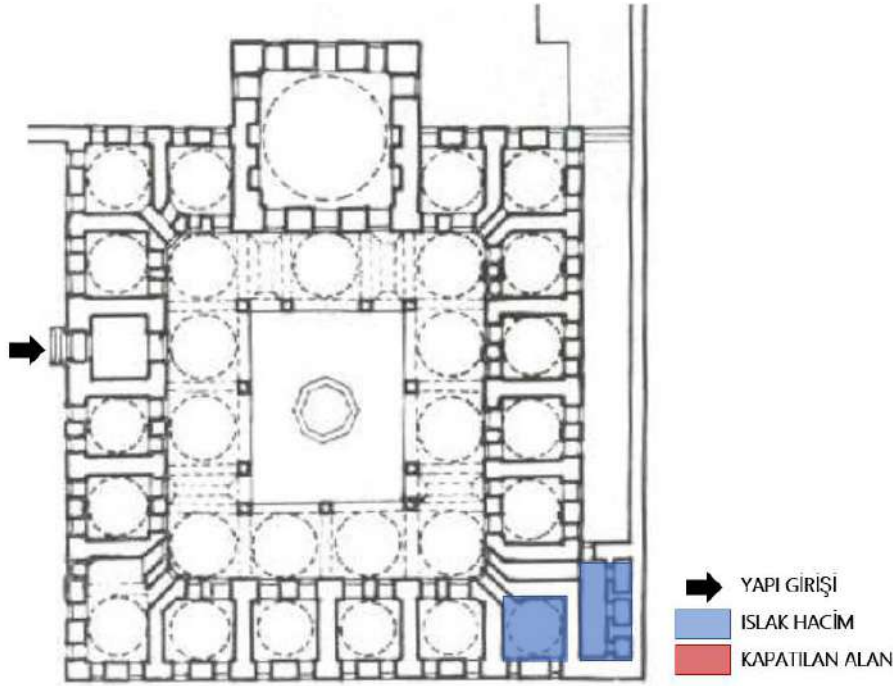
Şekil 3: Kılıç Ali Paşa Medresesi Planı (Ülgen, 1946)
